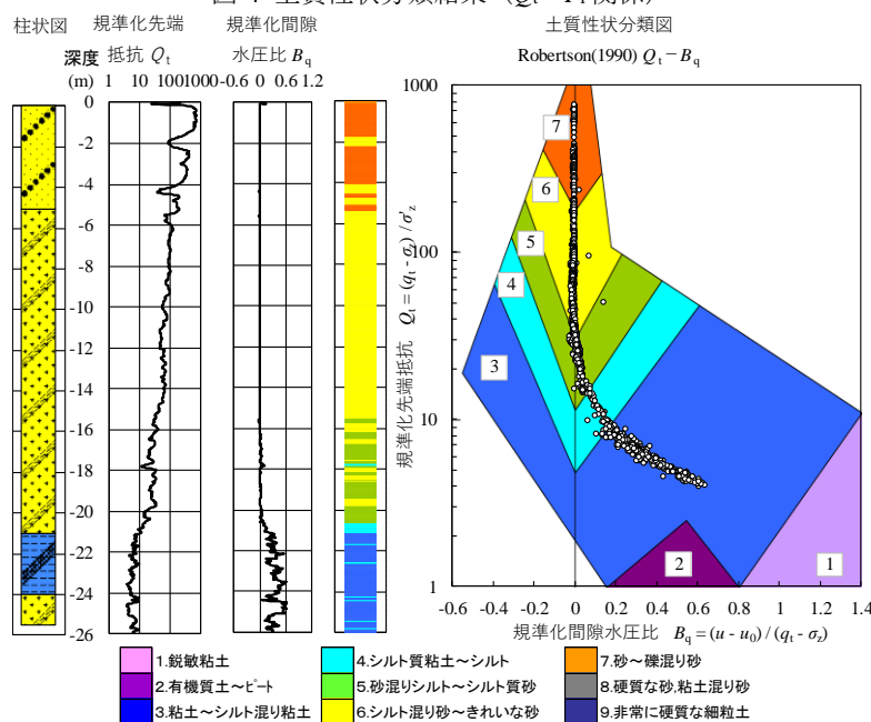
図-5 土質性状分類結果 ( Q_t-B_q 関係)
