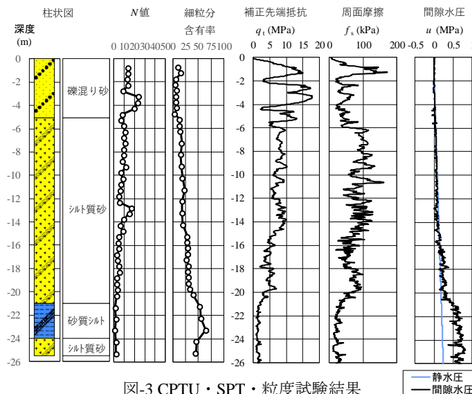
図-3 CPTU・SPT・粒度試験結果
