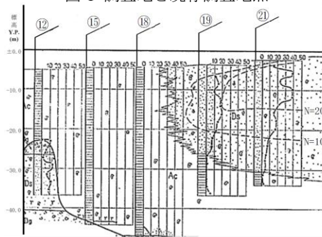
図-2 霞ヶ浦湖底想定断面図 ③
