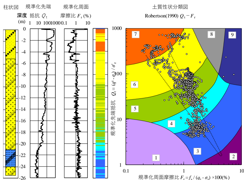
図-4 土質性状分類結果 ( Q_t-F_r 関係)
