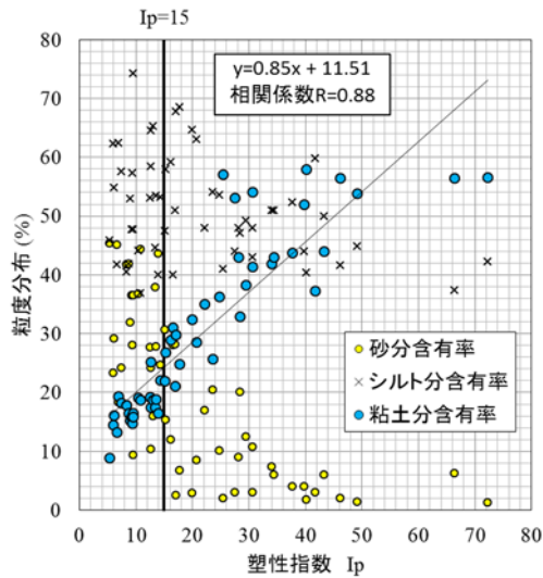
図-8 I_p と粒度分布の関係
