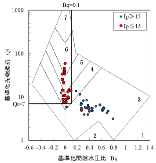
図-12 I_p の分布( Q_t \sim B_q )
