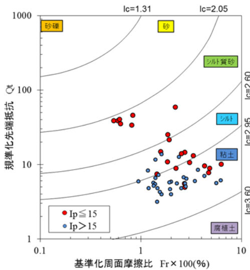
図-10 I_p の分布( Q_t \sim F_r )
