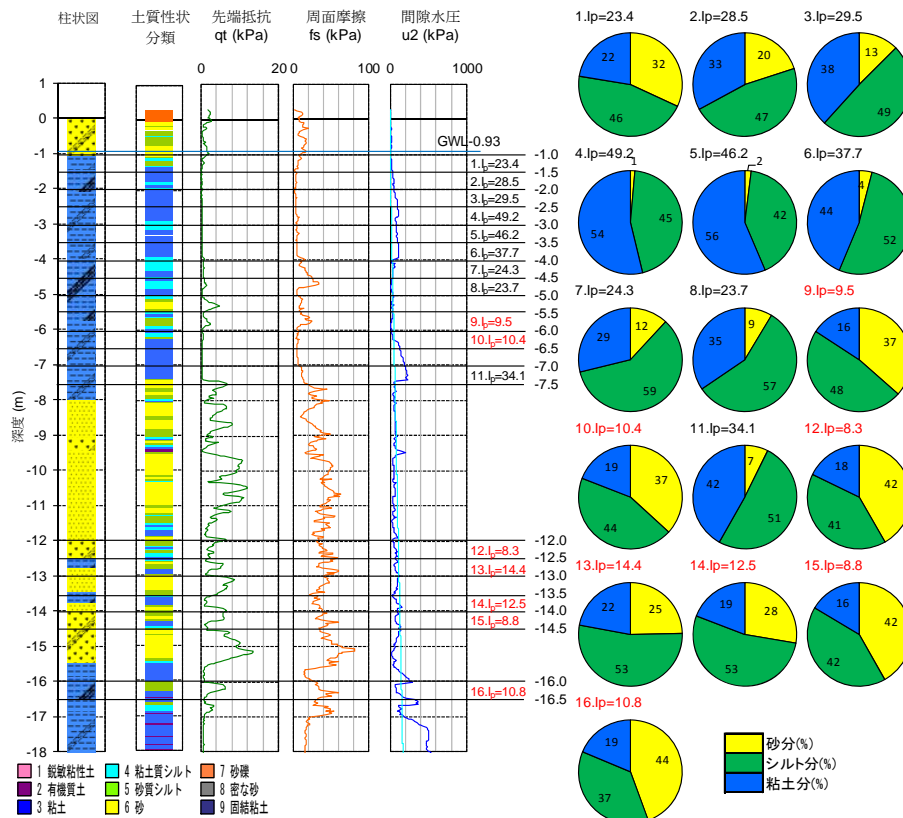
図-7 CPT 測定結果と粒度試験結果の対比の例 (浦安 3)
