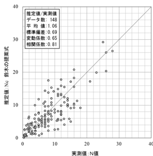
図-3 実測 N 値と推定 N_c の対比
