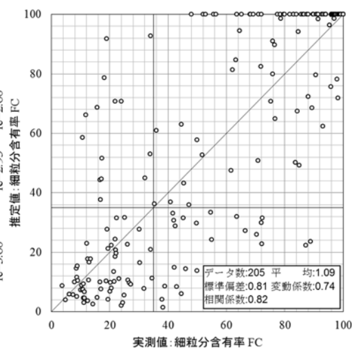
図-6 実測 FC と推定 FC の対比
