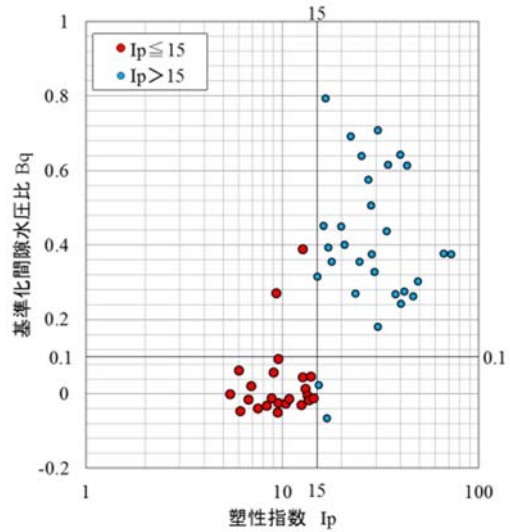
図-11 B_q と I_p の関係
