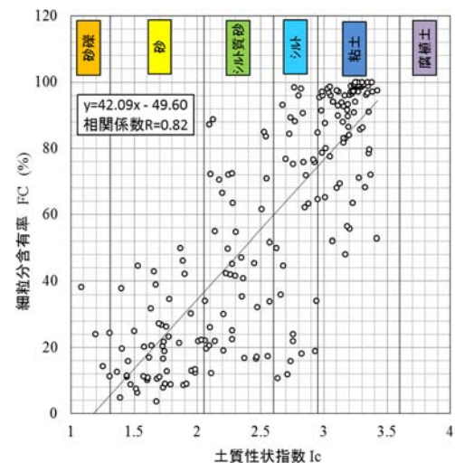
図-5 I_c と FC の関係
