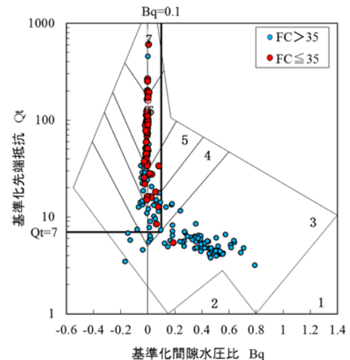
図-13 FC の分布( Q_t \sim B_q )
