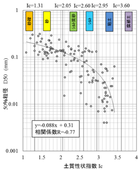
図-2 I_c と D_{50} の関係
