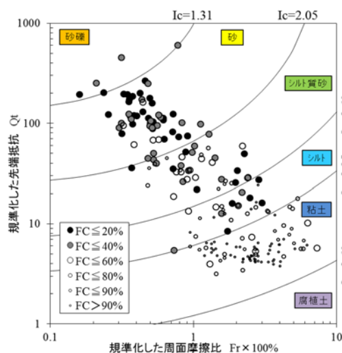
図-4 FC の分布
