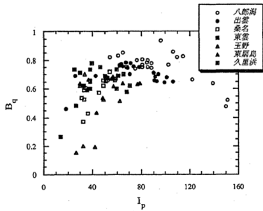
図-9 基準化間隙水圧と塑性指数の関係
