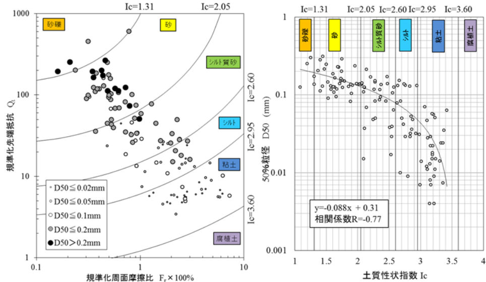
図-1 Q_t と F_r および I_c の関係と D_{50} の分布
